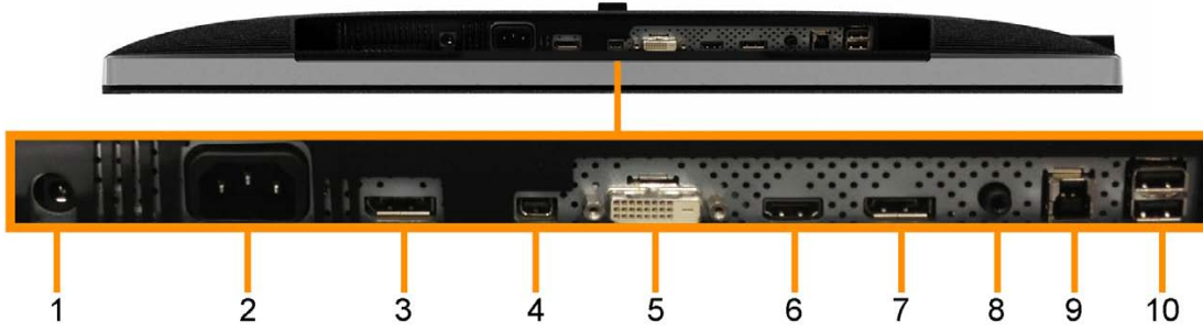
Alttan görünüm
